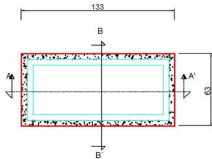
Vista planta
