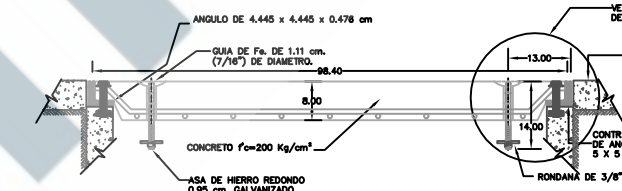
DETALLE TAPA: CORTE C-C?
