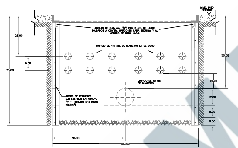
CORTE B-B?
