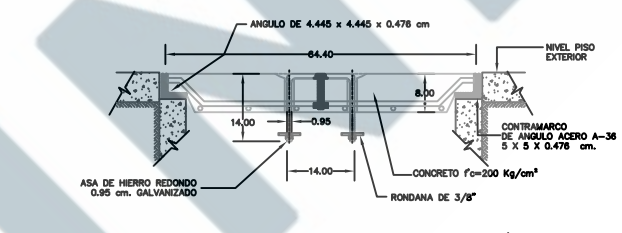
DETALLE TAPA: CORTE D-D?
