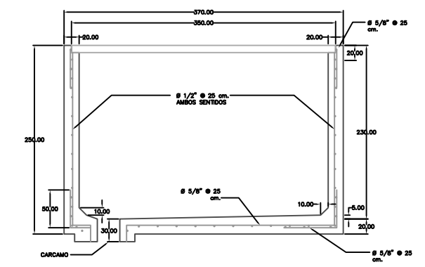
PARA NIVEL FREÁTICO BAJO SECCIÓN CORTE A-A'
