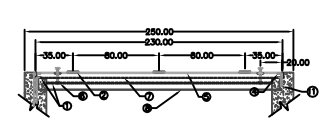
PLANTA SECCIÓN CORTE D-D'
