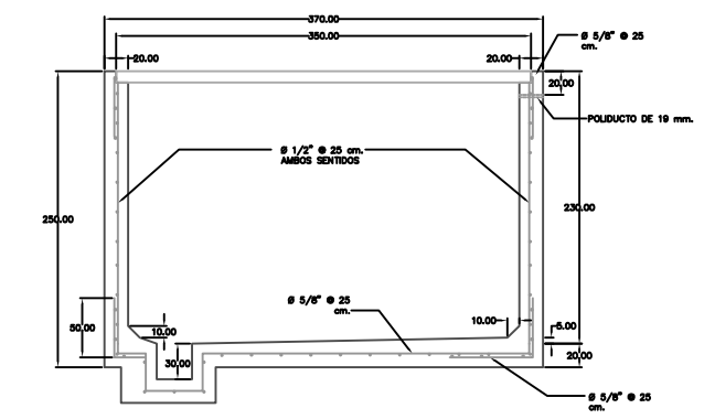
PARA NIVEL FREÁTICO ALTO SECCIÓN CORTE A-A'
