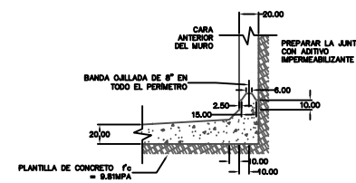
DETALLE 2
