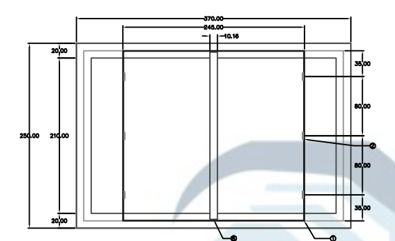
PLANTA MARCO Y BÓVEDA
