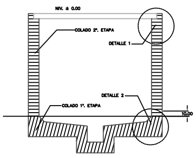
ETAPAS DE COLADO
