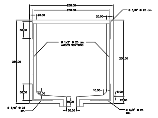
PARA NIVEL FREÁTICO BAJO SECCIÓN CORTE B-B'
