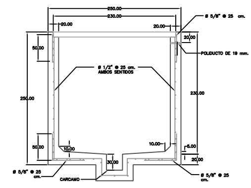
PARA NIVEL FREÁTICO ALTO SECCIÓN CORTE B-B'
