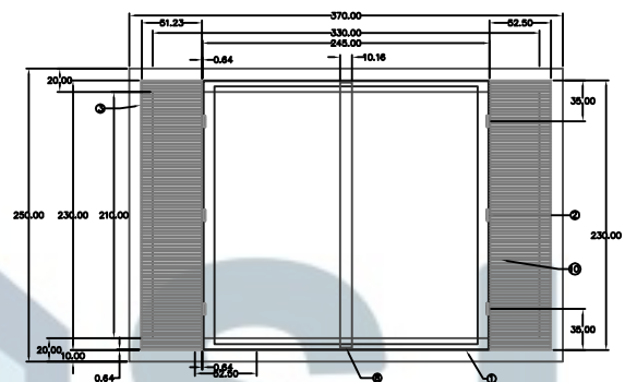
PLANTA MARCO, REFUERZOS Y REJILLA
