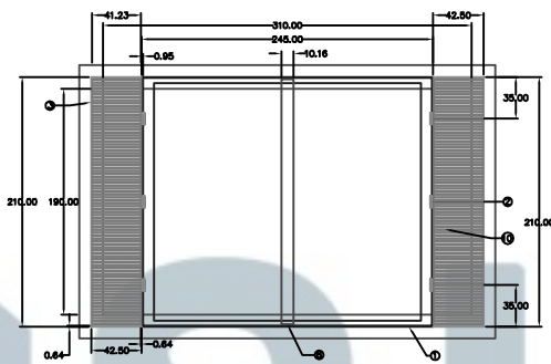
PLANTA MARCO, REFUERZOS Y REJILLA
