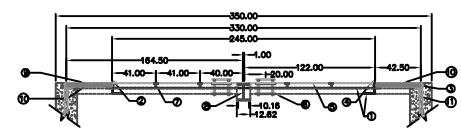
PLANTA SECCIÓN CORTE C-C'
